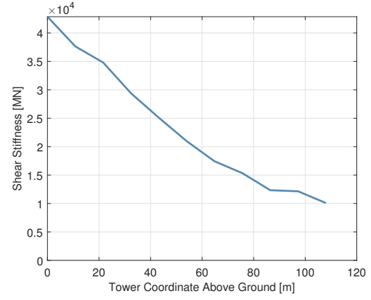
(d) Shear stiffness distribution
