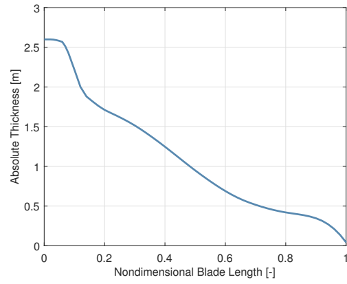
(d) Absolute thickness
