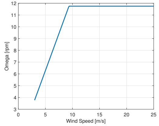
(d) Rotor speed
